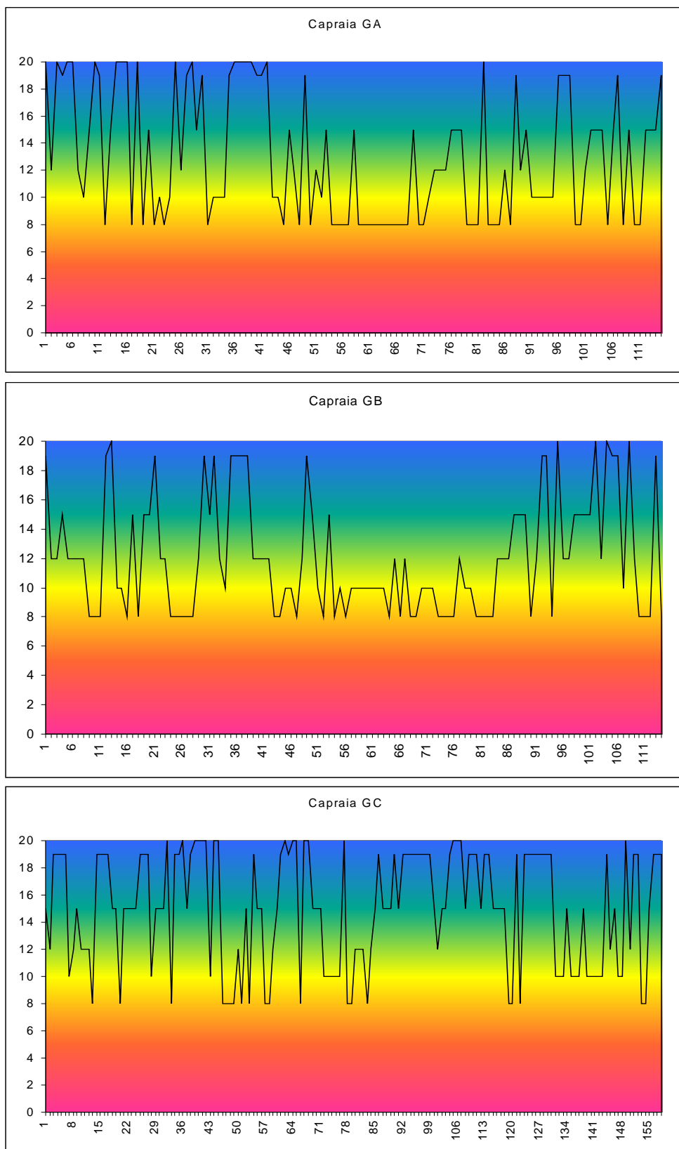
Figura 5.6 Rappresentazione grafica dei settori dell'Isola di Capraia (Arcipelago toscano).
