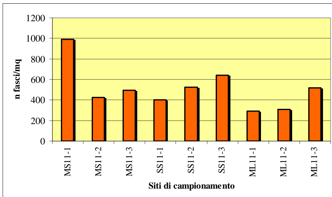
Figura 5.10. Densità dei fasci fogliari di Posidonia oceanica (in numero di fasci/m 2 ) rilevata presso le stazioni a 15 m di profondità dei diversi siti campionati nel 2012. MS = Isola di Montecristo(Arcipelago Toscano); ML = Mola-Elba sud (Arcipelago Toscano); SS = Porto Santo Stefano (Costa dell'Argentario).
