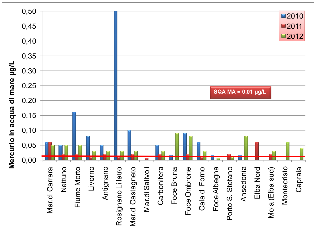
Figura 6.1 – Andamento della concentrazione di mercurio lungo la costa toscana triennio 2010-2012
